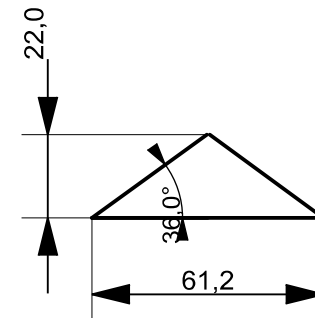
Dachstütze Profil 30x18 4 Stück gleiche Länge
