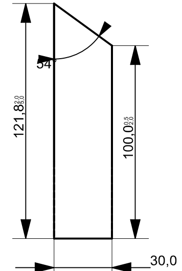
Dachstütze Profil 30x18 4 Stück gleiche Länge
