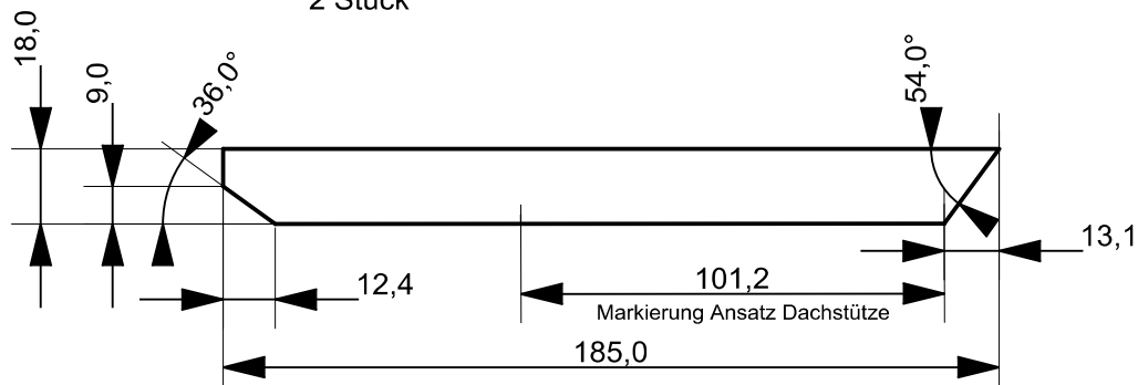
Dachpfette - Profil 18x18 4 Stück
